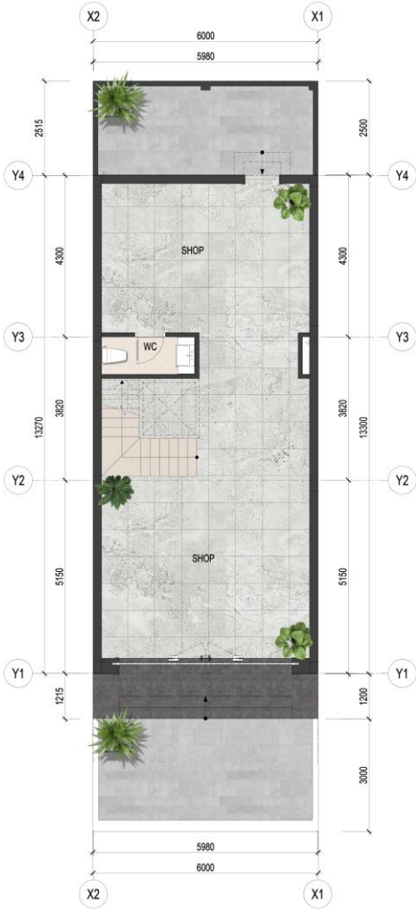
MẶT BẰNG TẦNG 1 ( S=79.8 M2 )
